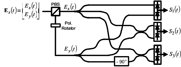
Fig. 3. Polarization-shift keying (PolSK) receiver.
